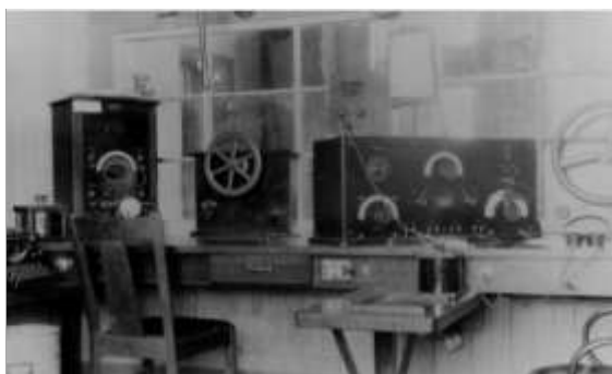
Рис. 4. Дуговой передатчик с радиоприёмником военно-морская радиостанция США на острове Русский (Владивосток) [3]. 1919 г.
