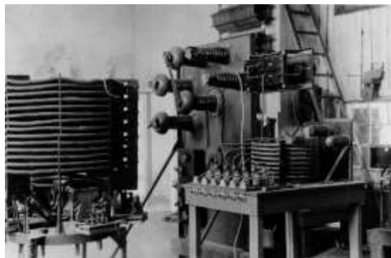
Рис. 5. Передающее оборудование военно-морской радиостанция США на острове Русский (Владивосток) [3]. 1919 г.
