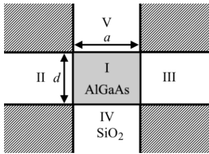
Рис. 1. Поперечное сечение исследуемых волноводных структур, где область I – сердцевина из AlGaAs с показателем преломления n_1 = 3.245 , область IV – подложка из SiO 2 с n_4 = 1.444 , области II, III, V – обкладка из воздуха с n_{2,3,5} = 1 или SiO 2 с n_{2,3,5} = 1.444 для полоскового и канального волноводов, соответственно
