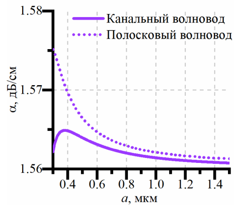
Рис. 3. Зависимость потерь на распространение от ширины сердцевин a в канальном и полосковом волноводах для моды основного типа E_0^x
