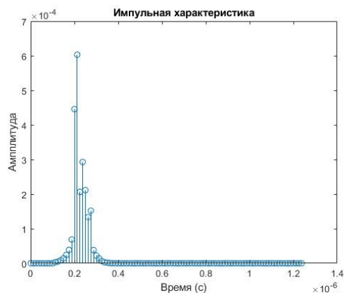
Рис. 2. Импульсная характеристика TGac
