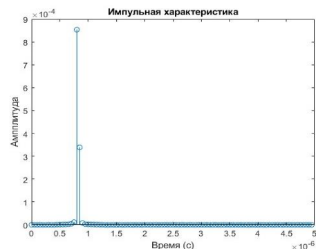
Рис. 1. Импульсная характеристика TGN
