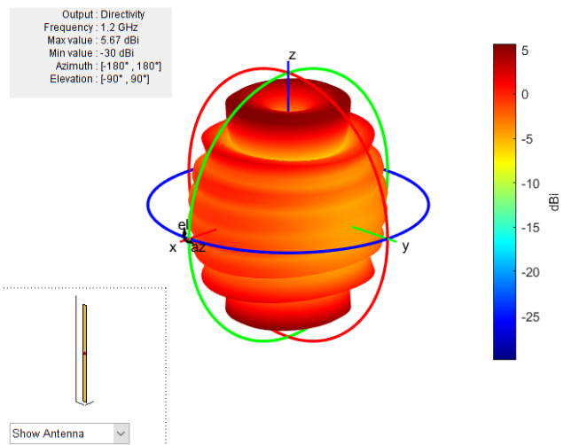
Рис. 3. 3D визуализация ДН дипольной антенны
