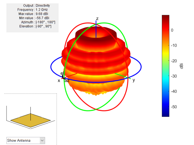
Рис. 4. 3D визуализация ДН штыревой антенны
