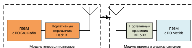
Рис. 1. Схема лабораторной установки
