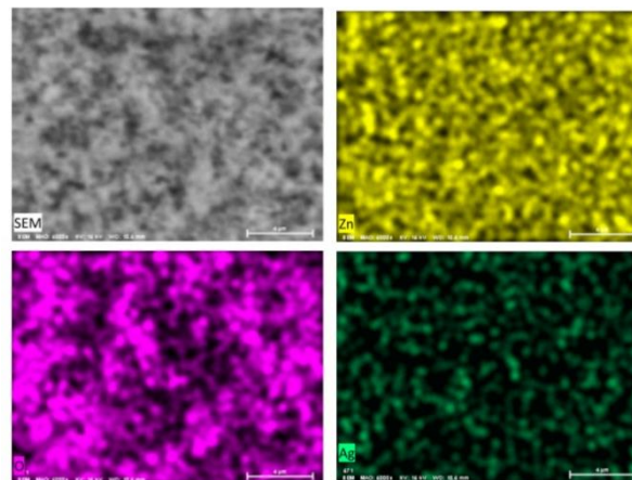
Рис. 3. Элементная карта ZnO/Ag-0,2: а) – СЭМ снимок поверхности; карта концентраций элементов: б) – Zn; в) – O; г) – Ag
