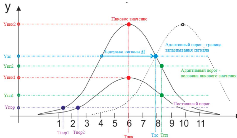
Рис. 1. Характеристическая кривая излучения
