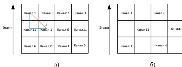
Рис. 3. Вертикальное расположение каналов для диапазона 2,4 ГГц
