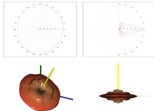
Рис. 5. Пример диаграммы направленности антенны точки доступа Wi-Fi с минимизацией излучения в вертикальной оси
