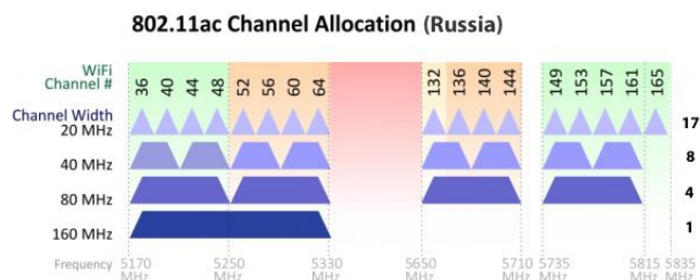
Рис. 1. Доступные каналы в частотном диапазоне 5 ГГц [5]
