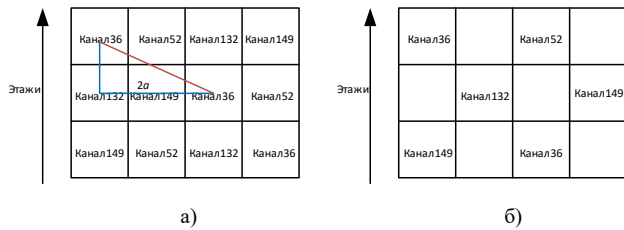
Рис. 4. Вертикальное расположение каналов для диапазона 5 ГГц, разрешенного для использования в Российской Федерации
