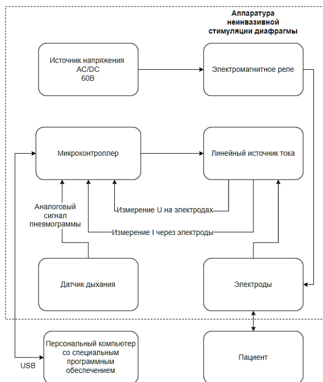
Рис. 5. Структурная схема аппарата неинвазивной стимуляции диафрагмы
