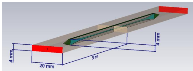
Рис. 1. Модель фазовращателя
