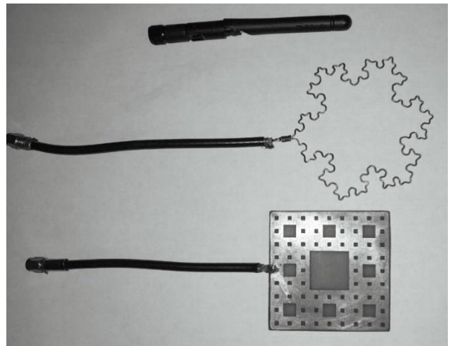
Рис. 5. Антенны. Сверху вниз: маленькая штыревая, «Снежинка Коха», «Ковёр Серпинского»
