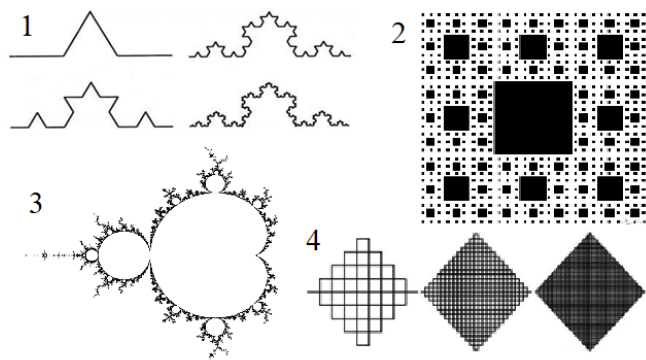
Рис. 1. Примеры фракталов
